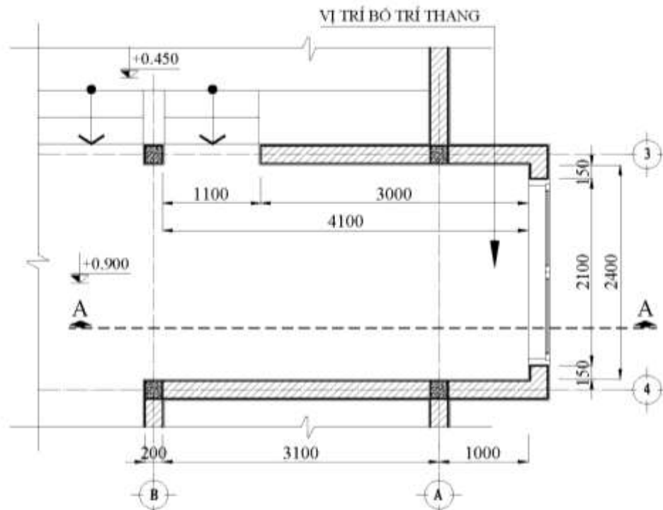
HÌNH 1: MB BỐ TRÍ THANG TÀNG TRỆT
