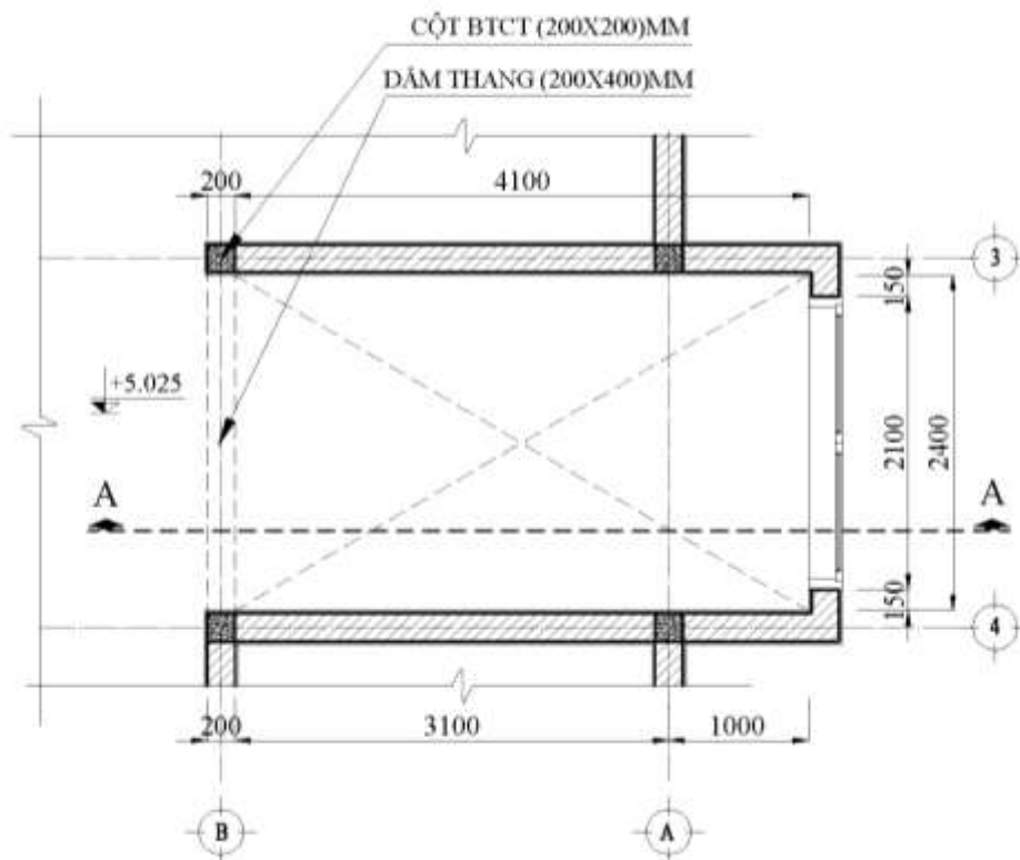
HÌNH 2: MB BỐ TRÍ THANG TÀNG LẦU
